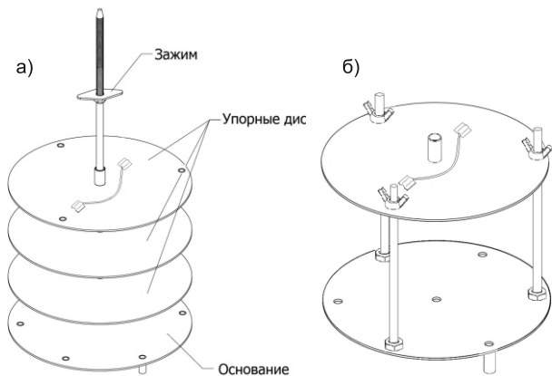
Рисунок 1. Кассета для автоклава: а) 1-ый вариант кассеты для 0,5; 0,7 и 1 л банок; б) 2-ой вариант кассеты для 1,5; 2 и 3 л банок.
